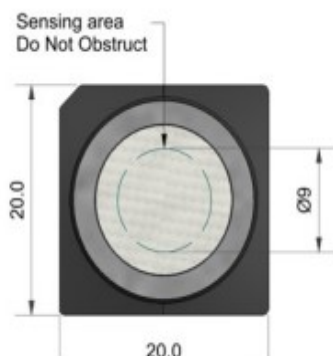
顶视图
